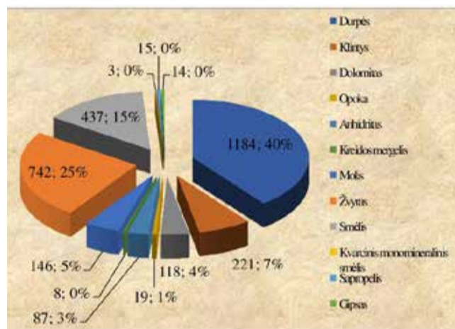
Detaliai išvalgytų Lietuvos naudingųjų iškasenų išteklių struktūra 2023 metų pabaigai, mln. kub.m
