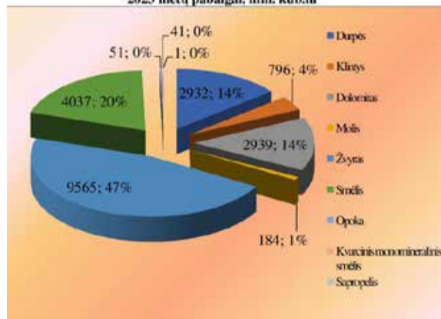
Naudingųjų iškasenų gavybos struktūra 2023 metais, tūkst. kub. m
